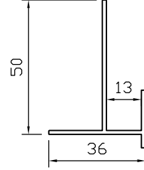
No: Y43381 Damlalık Profili
