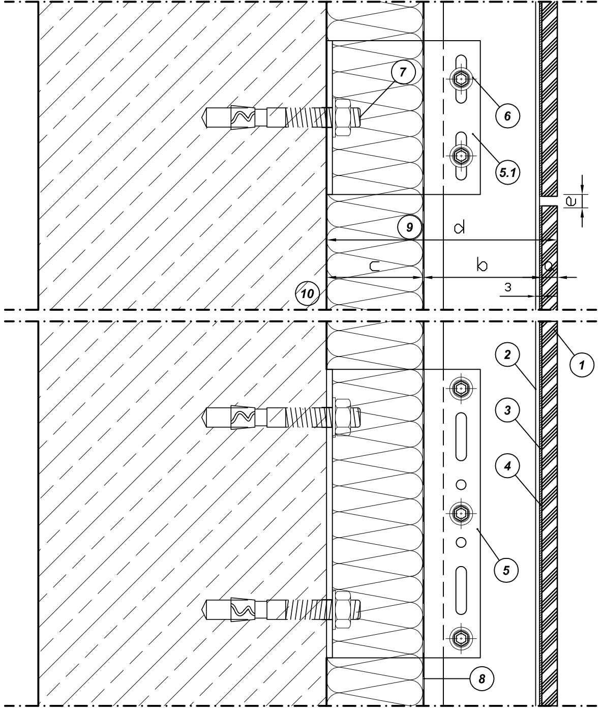
v.s.-1.1 DETAYI
