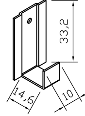
No: K1 Alt Klips
