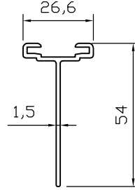
No: T43541 Tekli Profil 1,5mm
