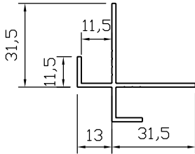
No: Y39422 Köşe Profili
