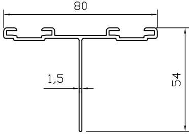
No: T41037 Çiftli Profil 80 lik 1,5mm
