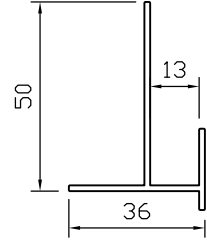
No: Y43381 Damlalık Profili
