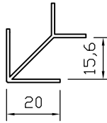
No: 10127 Köşe Profili max 11mm seramik
