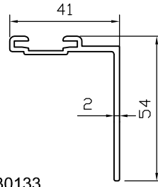
No: 30133 Tekli L Profil
