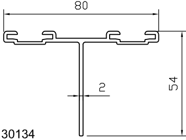
No: 30134 Çiftli Profil 80 lik
