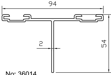
No: 36014 Çiftli Profil 94 lük
