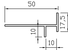
No: Y41047 Damlalık Profili
